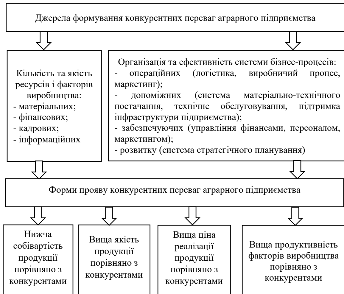
Рис. 1. Джерела та форми прояву конкурентних переваг аграрного підприємства
