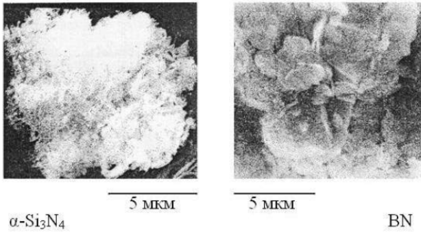
Рис. 6. Агломератні СВС-порошки
