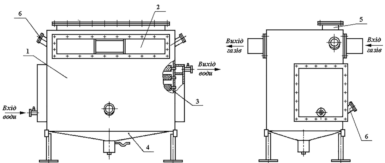
Рис. 1. Схема конденсаційного поверхневого теплоутилізатора:
