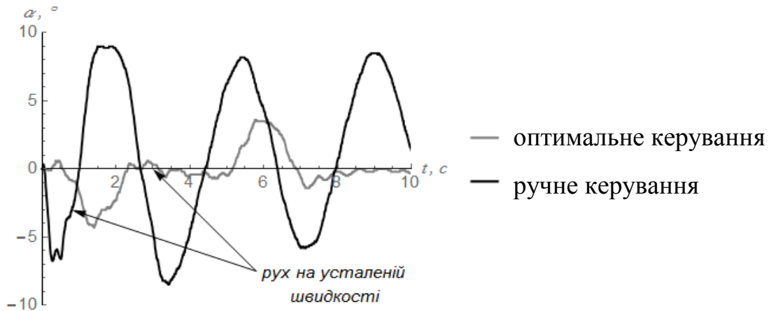
Рис. 3. Коливання вантажу відносно вертикалі при оптимальному та ручному керуванні
