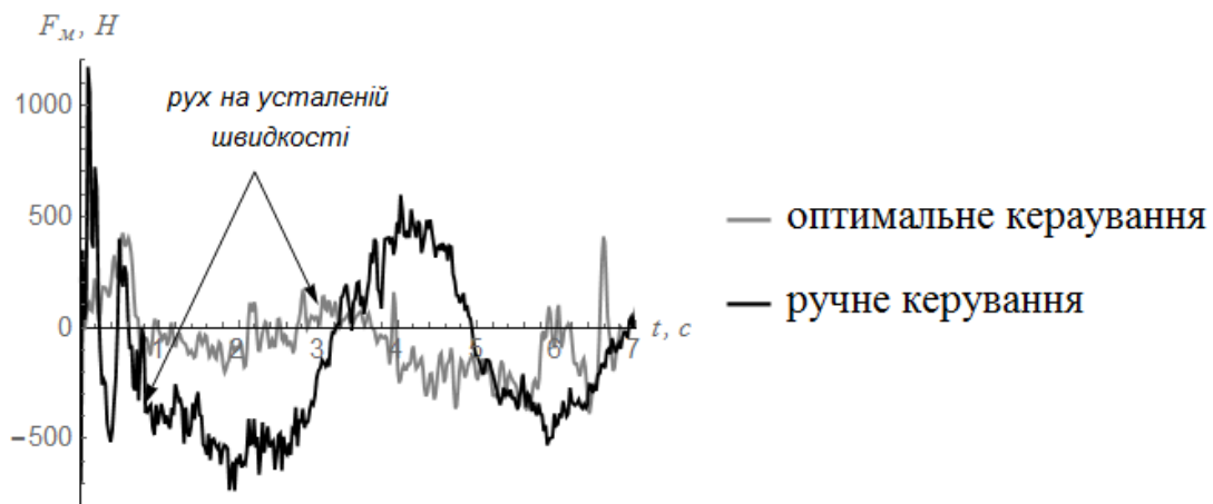
Рис. 2. Зусилля, що діє в мостовій балці крана у горизонтальній площині під час переміщення при оптимальному та ручному керуванні.
