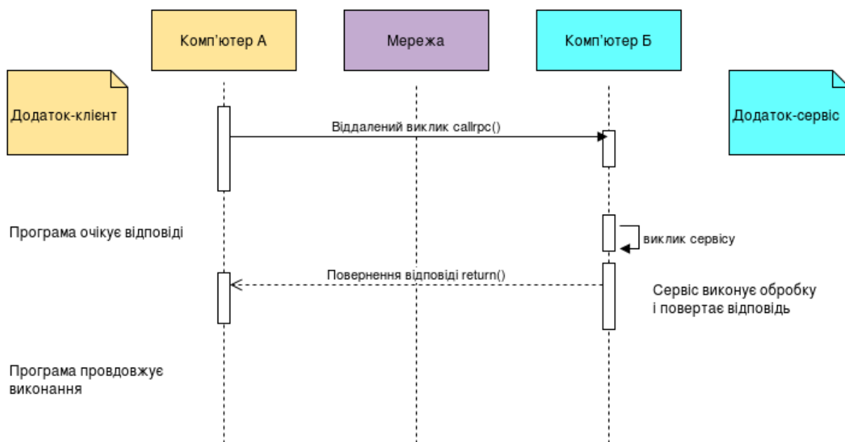
Рисунок 1. – Діаграма послідовності RPC
