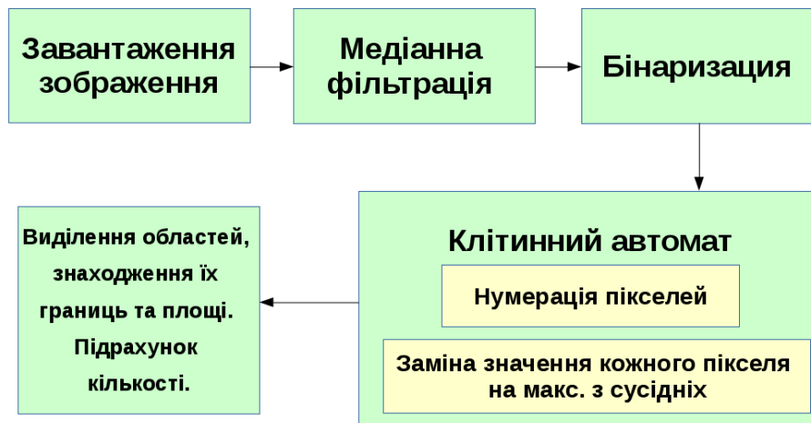
Рисунок 2 – Алгоритм роботи створеного програмного продукту
